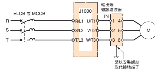
連接圖
