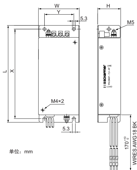
图 D.7 EMC 噪音滤波器的外形尺寸
