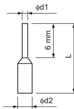
图 3.12 棒端子的外形尺寸图
