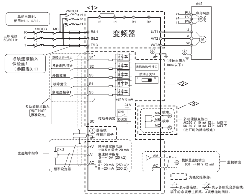
图 D.2 符合低电压指令的相互接线示例
