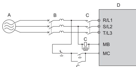
A - 三相 AC200 ~ 240 V 50/60 Hz 单相 AC200 ~ 240 V 50/60 Hz B - MCCB C - MC D - 变频器
