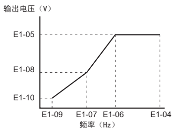
图 5.11 V/f 曲线图
