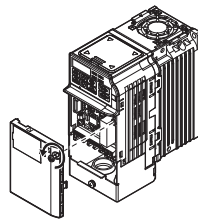
图 8.11 前外罩的拆卸方法
