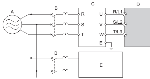
A - 电源 B - MCCB C - 输入侧（一次侧）噪音滤波器 型号：LNFD-□□ D - 变频器 E - 其它控制设备
