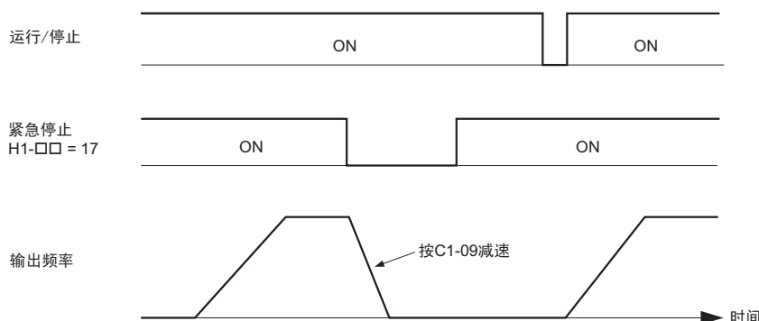
图 5.16 紧急停止的时序图
