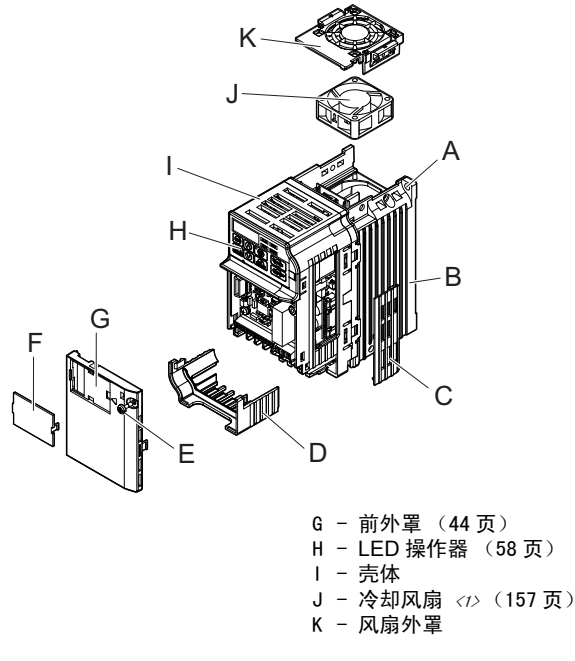
图 1.2 柜内安装型变频器各部分名称 CIMR-J□2A0006B
