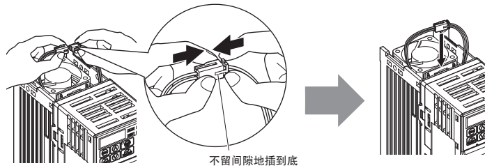
图 7.3 中转插头
