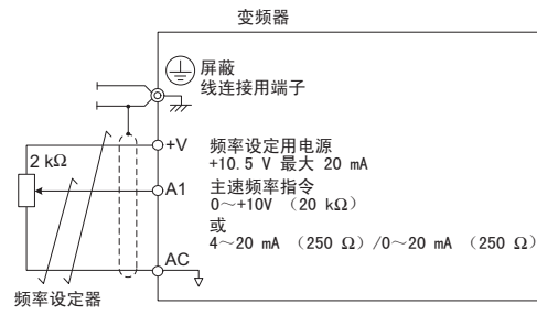
图 3.15 来自控制回路端子的频率指令
