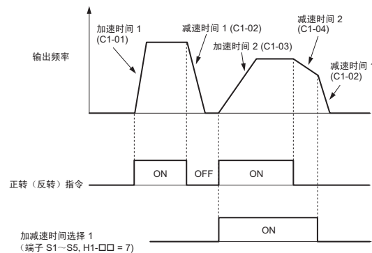
图 5.3 加减速时间的时序图
