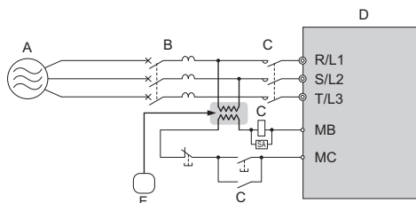
A - 三相 AC380 ~ 480 V 50/60 Hz B - MCCB C - MC D - 变频器 E - 400/200 V 变压器
