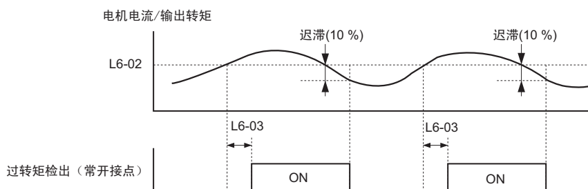
图 5.36 过转矩检出的时序图
