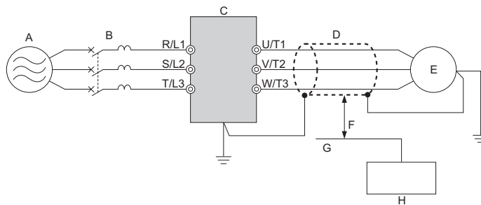
A - 电源 B - MCCB C - 变频器 D - 带屏蔽的电机电缆 E - 电机 F - 离开 30cm 以上 G - 信号线 H - 控制设备
