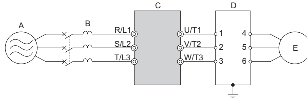
A - 电源 B - MCCB C - 变频器 D - 输出侧（二次侧）噪音滤波器 E - 电机
