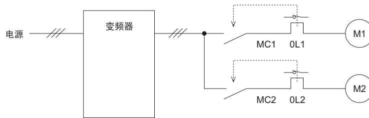
MC1, MC2...电磁接触器 OL1, OL2...热继电器
