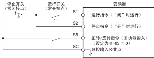
图 3.2 3 线制顺控
