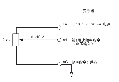
图 5.1 第 1 段速频率指令的电压输入
