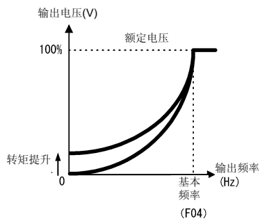
2 次方递减转矩特性 (F37=0)
