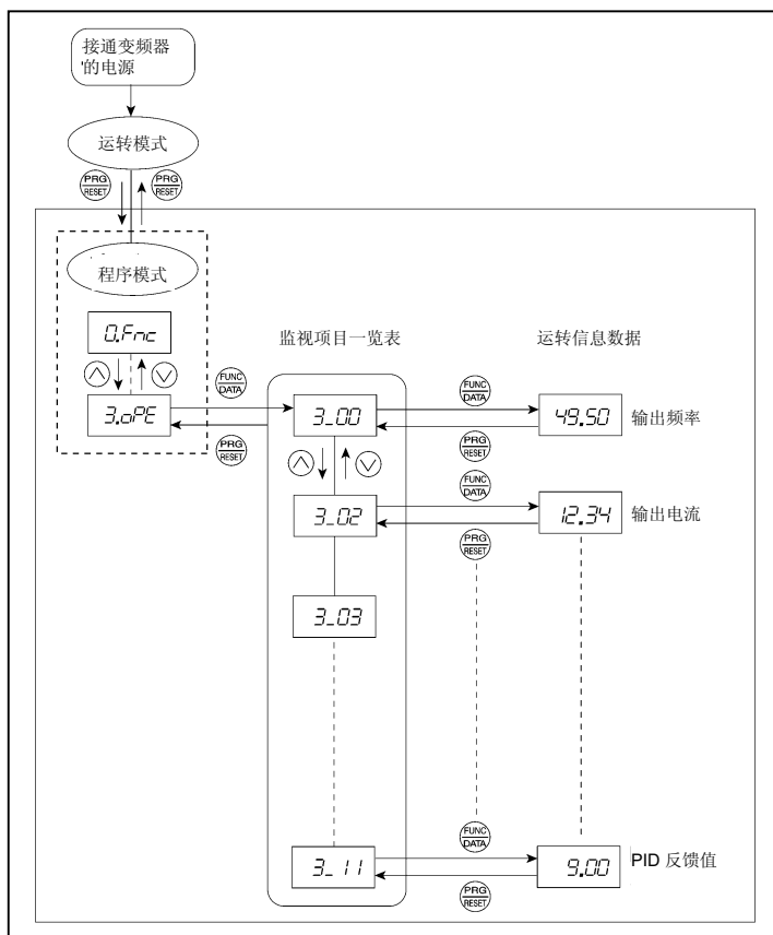
图 3.8 「运转监视」的菜单转换图
