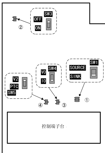
图 2.28 各种开关的位置
