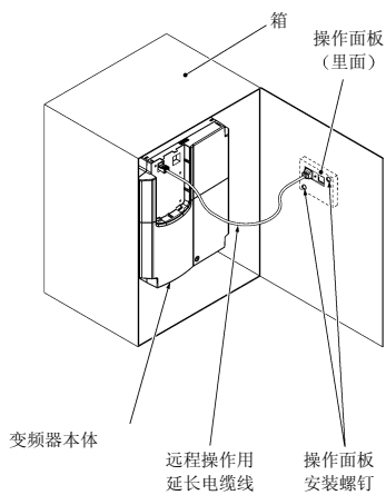
图 2.29 操作面板安装在控制柜内时
