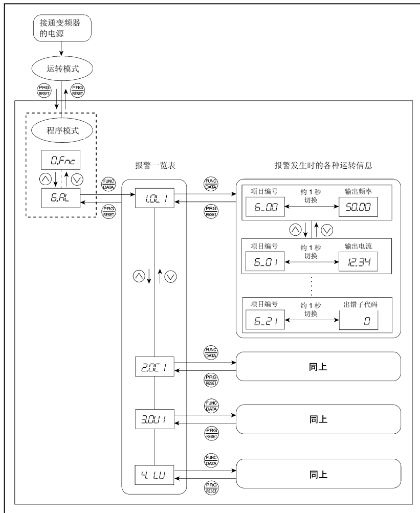
图 3.11 「报警信息」的菜单转换图
