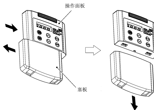
图 2.32 远程操作时的操作面板的分离和安装
