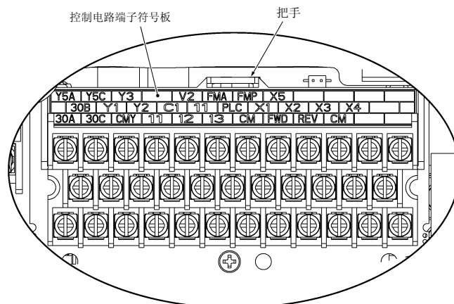
图 2.27 关闭控制电路端子符号板时
