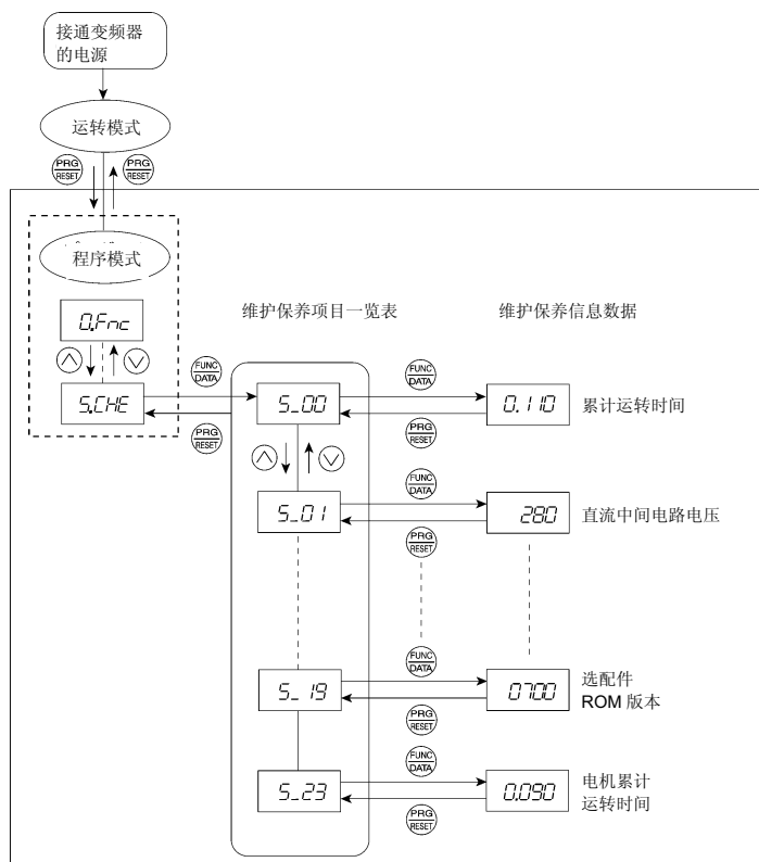
图 3.10 「维护保养信息」的菜单转换图
