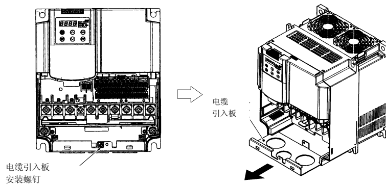
图 2.10 电缆引入板的拆除(FRN 15F1S-2J)
