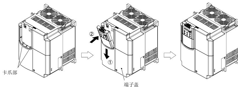
图 2.35 操作面板的安装
