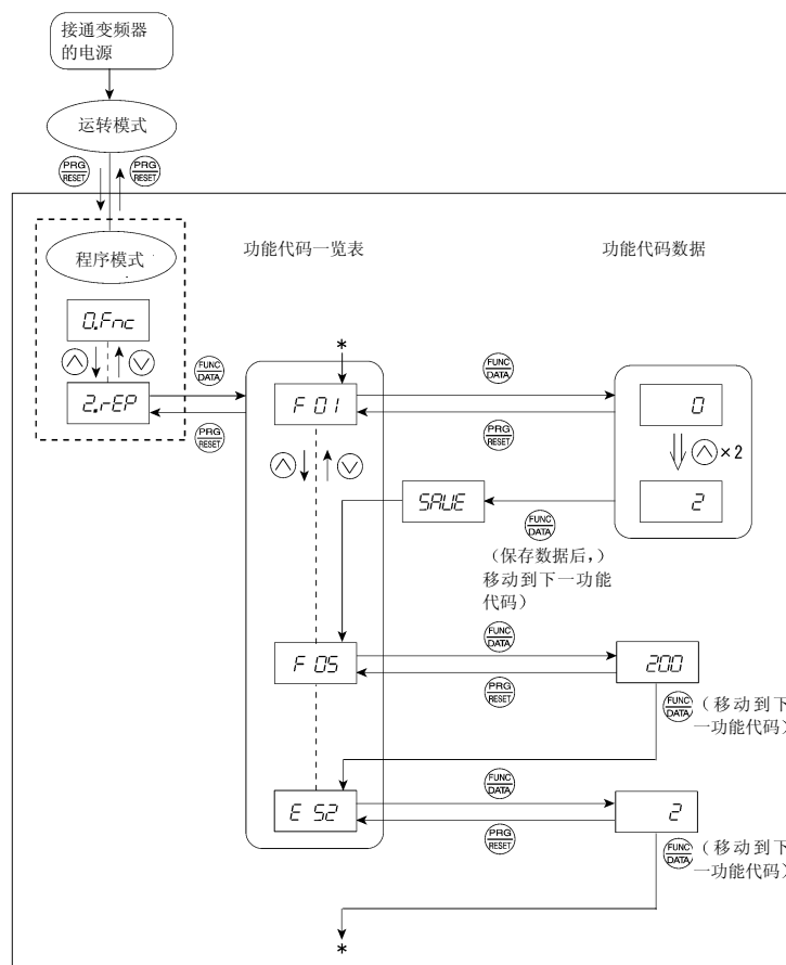
图 3.7 「数据确认」的菜单转换图（只更改 F01、F05、E52 时）
