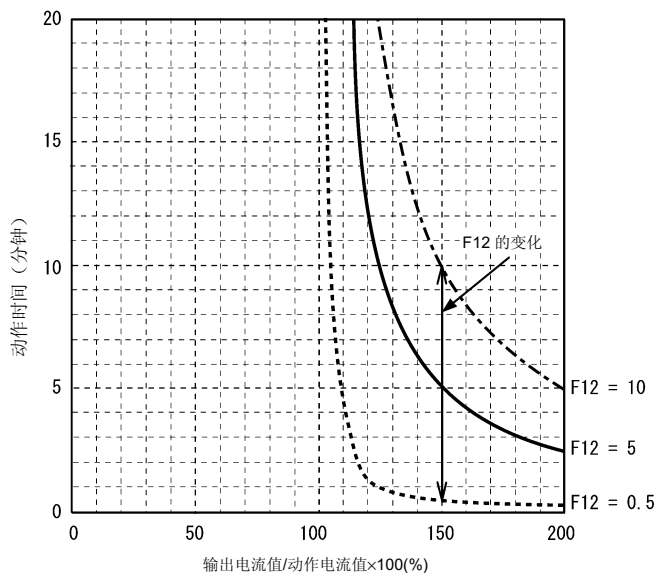
<电流-动作时间特性例>
