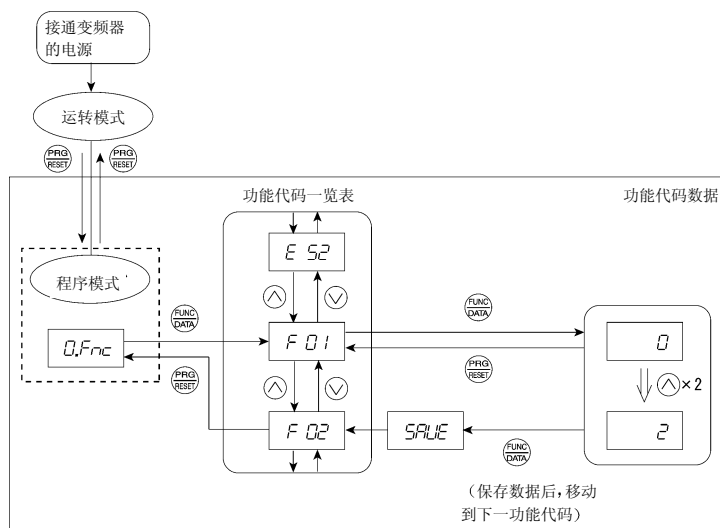
图 3.5 功能代码数据的更改顺序
