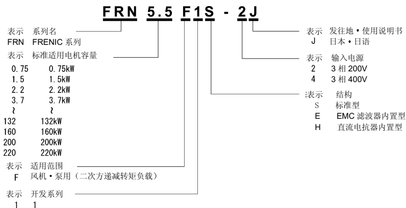
图 1.1 铭牌
