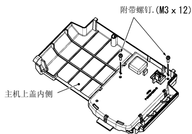
图 2.5 操作面板的固定
