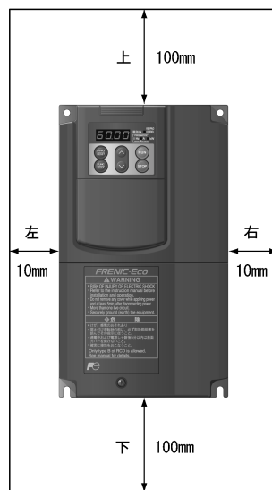
图 2.1 安装方向 (5.5kW 以下可以横向紧密安装)
