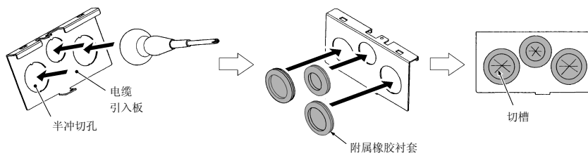
图 2.11 半冲切孔的打开方法和橡胶衬套的安装
