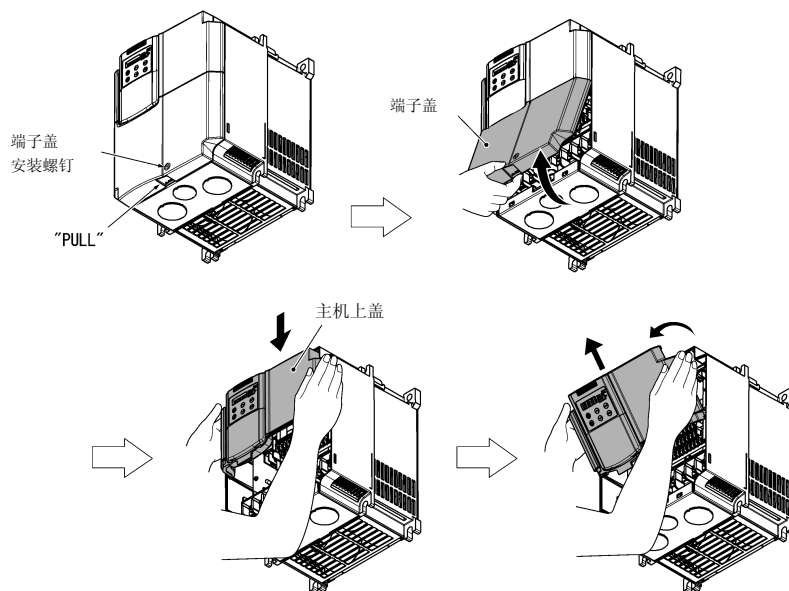
图 2.6 盖的拆除 (FRN15F1S-2J)
