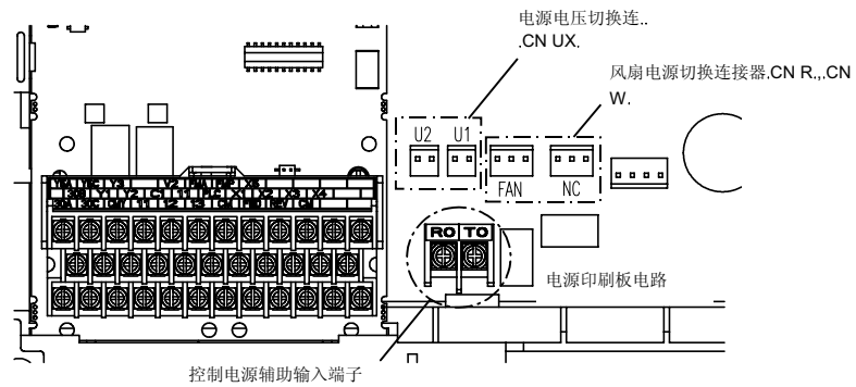
图 2.14 切换连接器的配置
