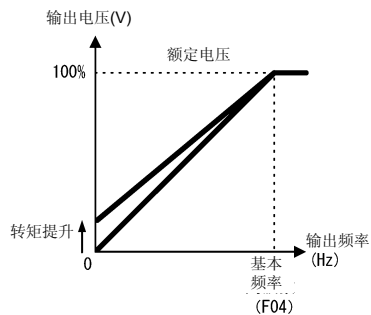
直线 V/f 特性 (F37=1)
