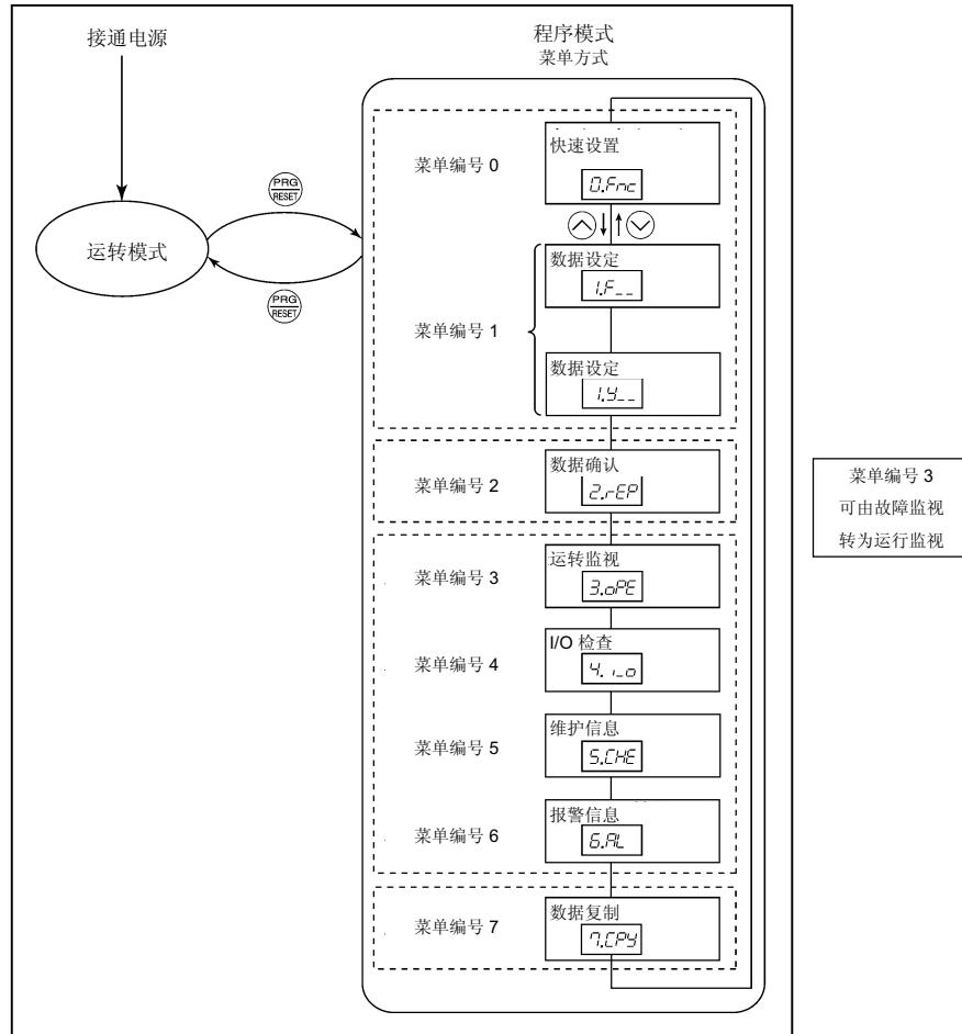
图 3.3 「程序模式」的菜单转换图
