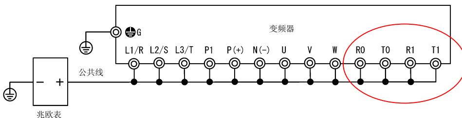
图 7.2 绝缘电阻测试
