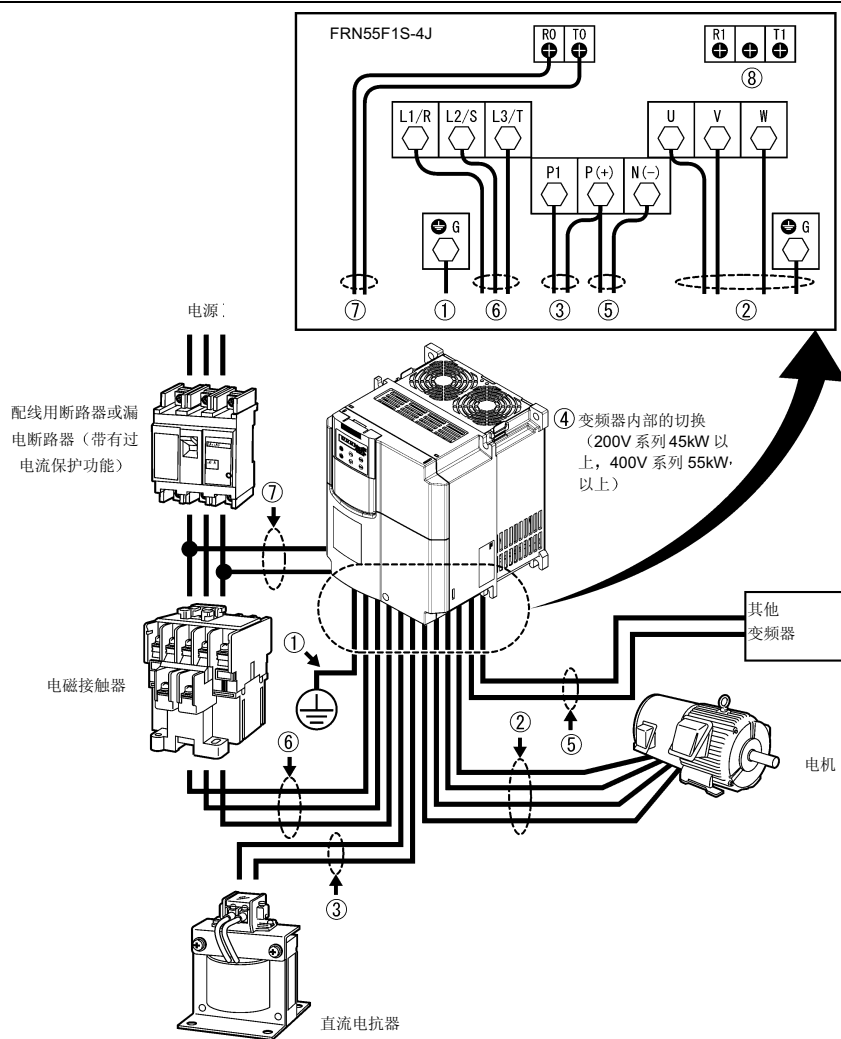
图 2.12 与设备的配线顺序
