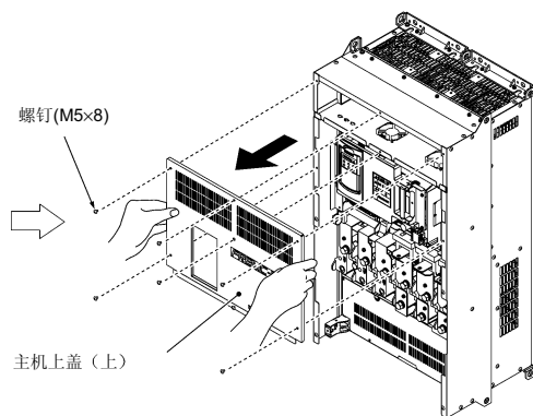
图 2.9 盖的拆除·安装 (FRN220F1S-4J)
