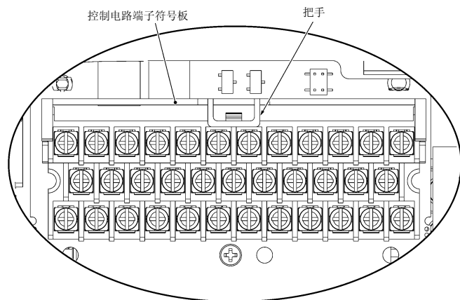
图 2.26 打开控制电路端子符号板时
