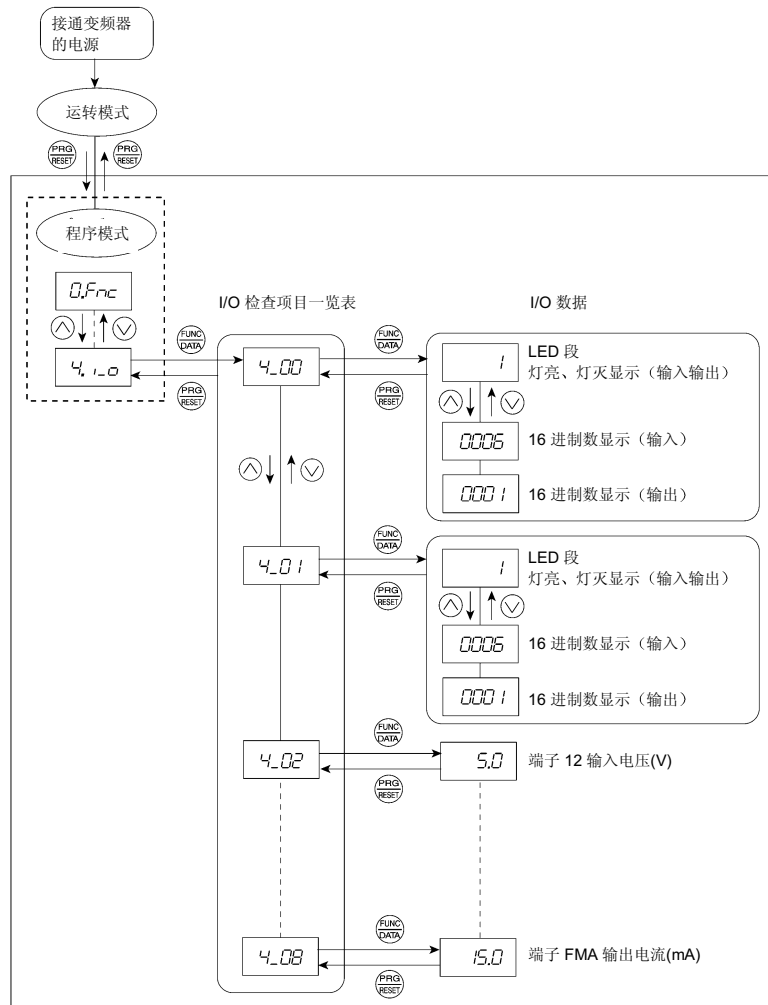
图 3.9 「I/O 检查」的菜单转换图
