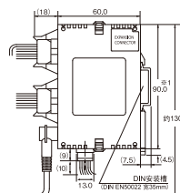
＜布线时参考尺寸＞
