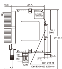
＜布线时参考尺寸＞
