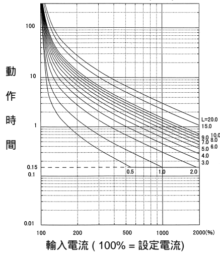
強反時限特性曲線( VI )
