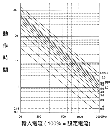
I 2 t特性曲線
