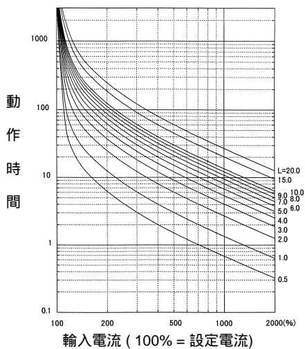
長反時限特性曲線( LT )
